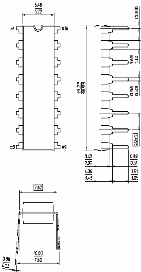
DIP16 外形尺寸图
