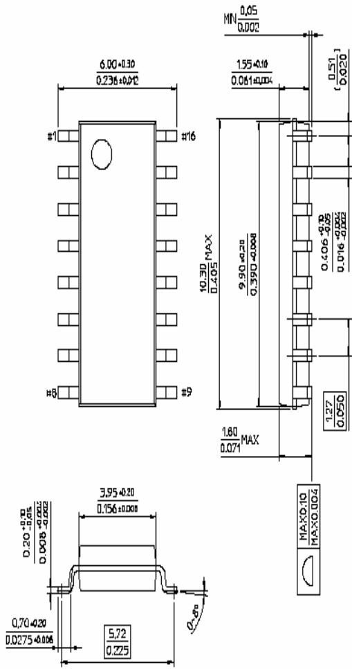
SOP16 外形尺寸图
